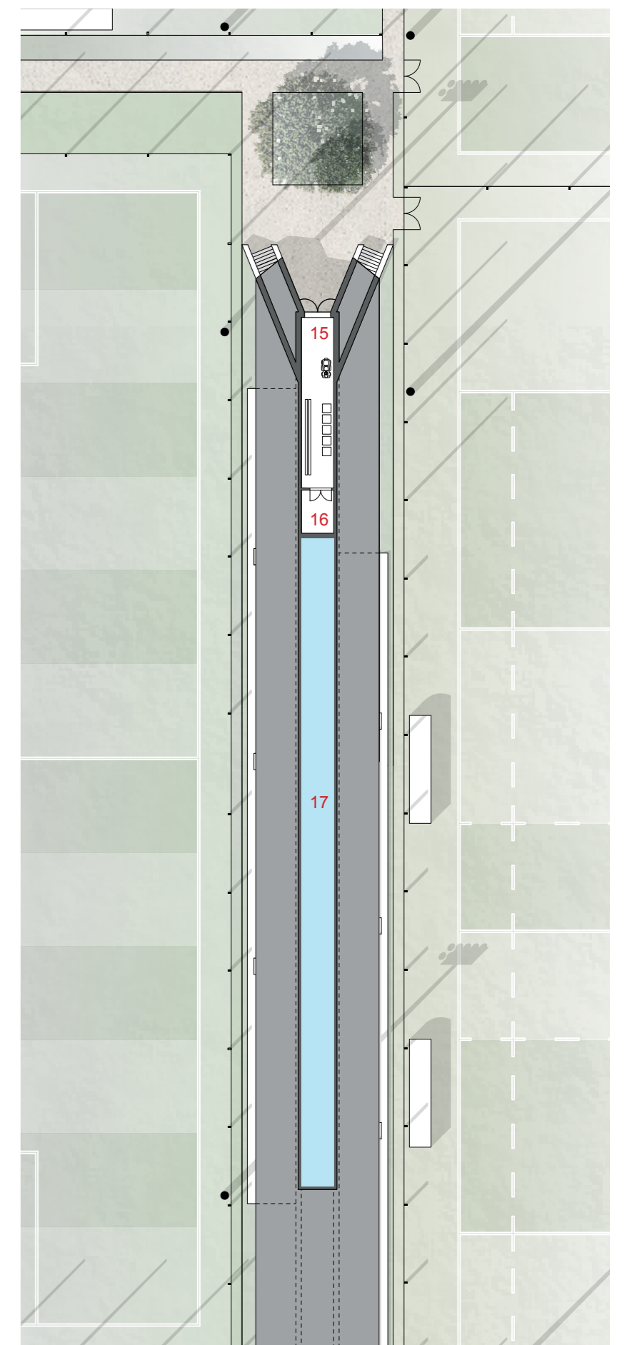
PIANTA SPAZI SOTTO LE TRIBUNE - SCALA 1:500
